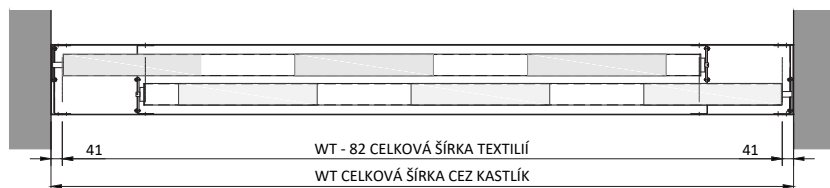
PÔDORYS - TYP AT-H-E
